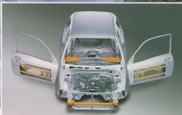
Podwójne belki w drzwiach i wzmocnienie frontu nadwozia to efekt wielu intensywnych testów, których wyniki ustaliły właściwą dla przyszłej Europy konstrukcję karoserii
